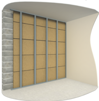
Figure 4.1 - Pose de l'ossature métallique (montants M48 doublés et rails R48) et Insertion des panneaux ISONAT FLEX (40 ou 100 mm) derrière l'ossature métallique
