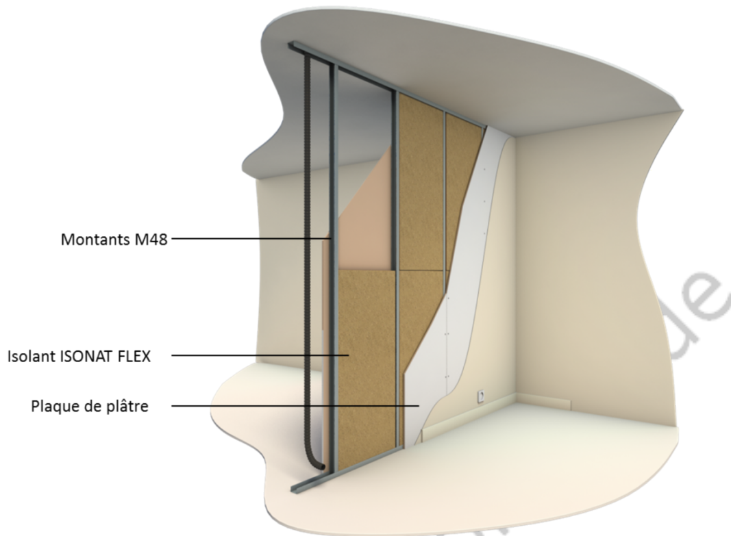
Figure 1 - Réalisation d'une cloison sur ossature métallique avec montants M48 simples (ISONAT FLEX en 40 mm)
