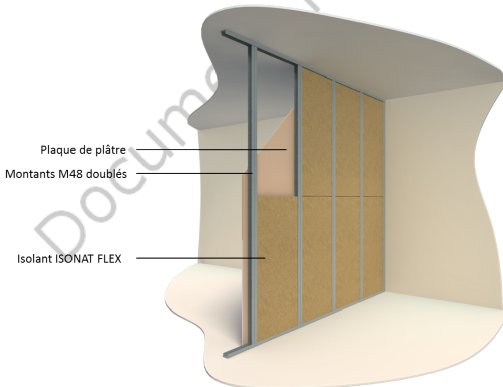
Figure 2 - Réalisation d'une cloison sur ossature métallique avec montants M48 doublés (ISONAT FLEX en 40mm)
