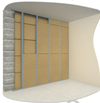
Figure 4.2 - Insertion de la 2 e couche ISONAT FLEX (40 mm) entre montants M48
