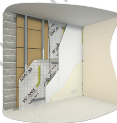
Figure 4.3 - Mise en place des profilés métalliques Stilmob et des gaines électriques et Pose des plaques de plâtre
