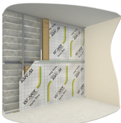
Figure 3.3 - Mise en place de la membrane pare-vapeur Vario® Xtra sur l'ossature métallique à l'aide de double face
