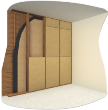
Figure 5.1 - Pose des isolants ISONAT FLEX entre montants bois
