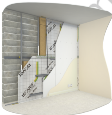
Figure 3.5 - Pose des plaques de plâtre
