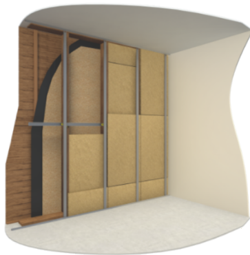
Figure 5.3 - Pose des lisses hautes et basses, et celles des fourrures métalliques verticales et de la seconde couche d'isolant entre fourrures
