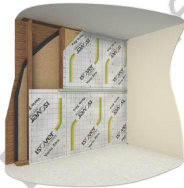
Figure 5.2 bis : Variante de pose de la membrane Vario® Xtra via agrafage sur montants bois et une seule couche d'isolant
