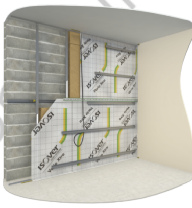
Figure 3.4 - Mise en place des profilés métalliques Stimob et passage des gaines électriques
