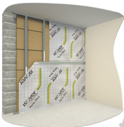
Figure 4.3 - Mise en place de la membrane pare-vapeur Vario® Xtra sur l'ossature métallique à l'aide de double face
