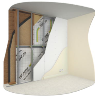
Figure 5.3 bis - Pose de la fourrure intermédiaire et des appuis Optima2 clipsés. Pose des fourrures métalliques verticales puis celle du parement de finition
