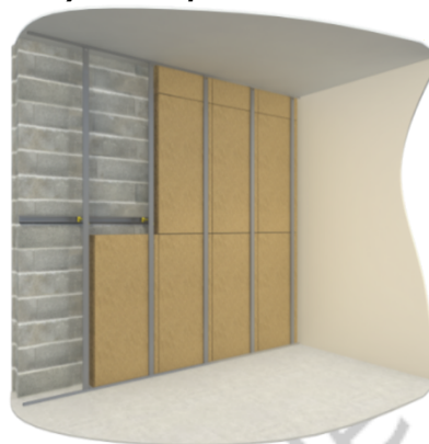
Figure 3.2 - Insertion des panneaux ISONAT FLEX derrière l'ossature métallique
