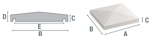
WCP38 / WCP48
